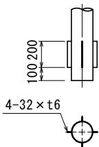
支柱下部詳細図 S=1:20
