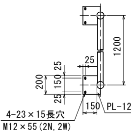
標識板取付金具詳細図 S=1:20
