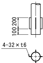
支柱下部詳細図 S=1:20
