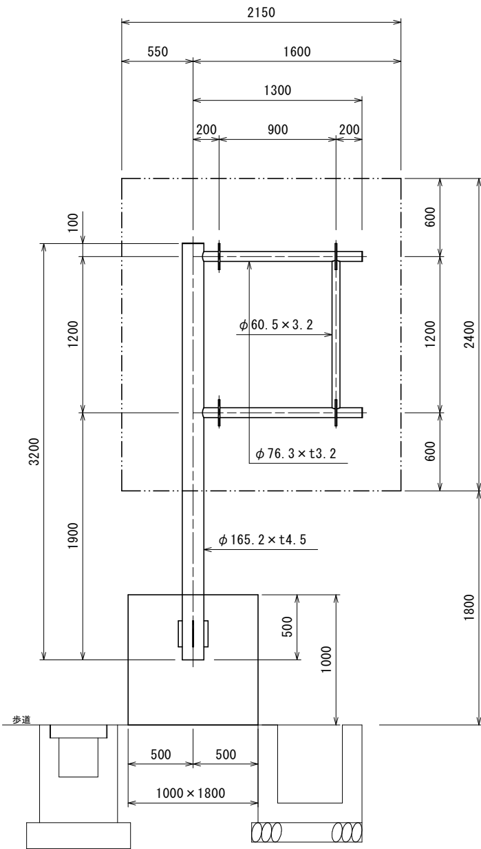
支柱外形図 S=1:20
